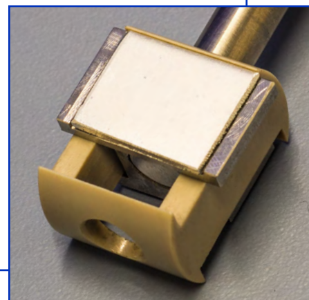
Магнитная система позиционирования твёрдых образцов
